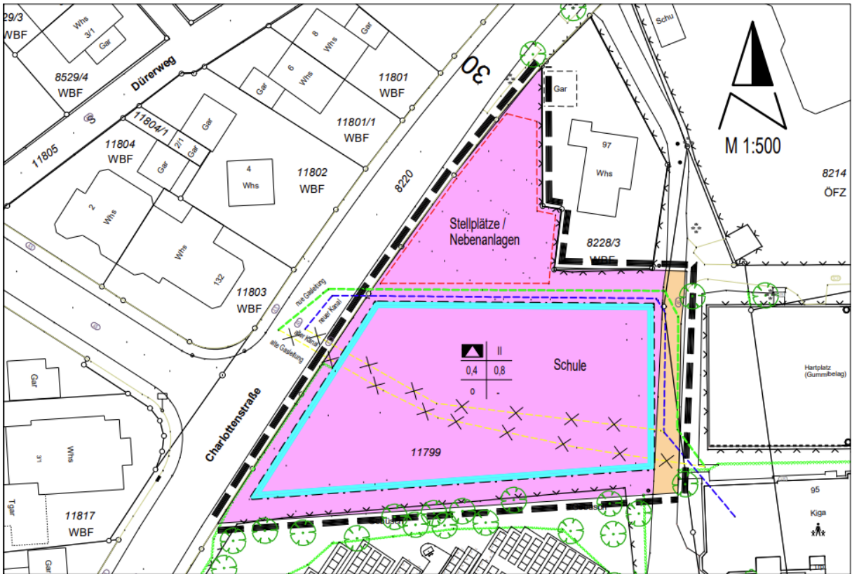
Vorentwurf Planzeichnung
